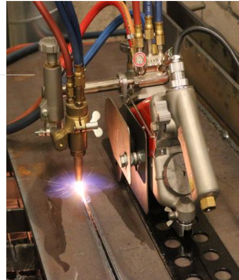
Führungsschiene für gerade Schnitte
